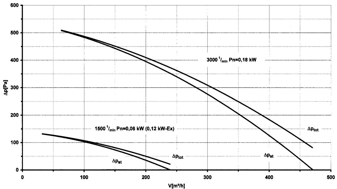
Kennlinie HF-Dv 110+
